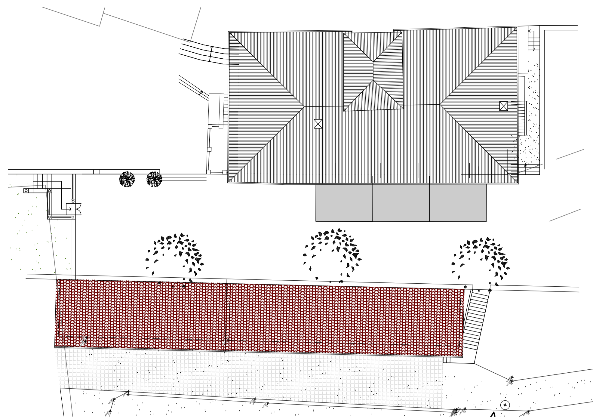
PLANIMETRIA - STATO DI FATTO SCALA 1:100
