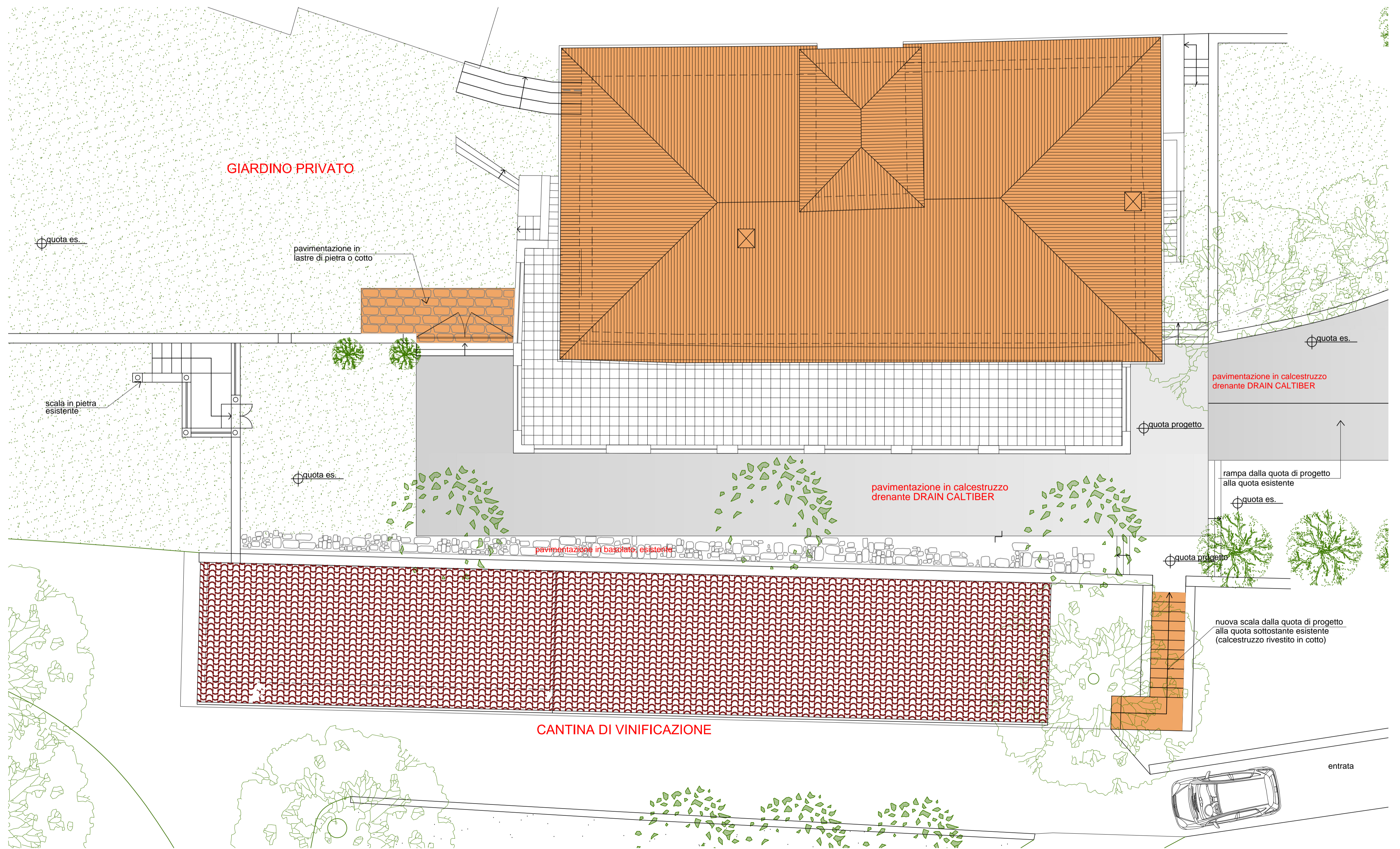
PLANIMETRIA SCALA 1:100
