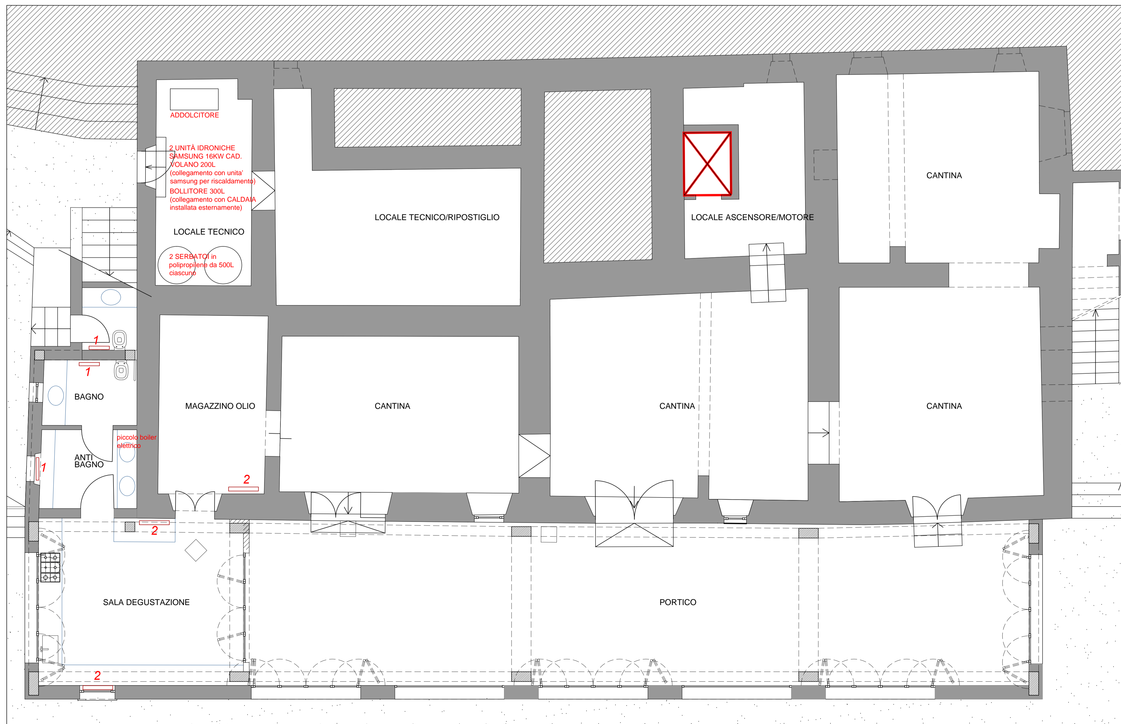
PLANIMETRIA - POSIZIONE SCHEMATICA DI TRE TUBAZIONI IN ACCIAIO DIAM. 10-12 INTERRATE DI COLLEGAMENTO TRA LA CANTINA DELLA VINIFICAZIONE E LA CANTINA DI CONSERVAZIONE SCALA 1:200
