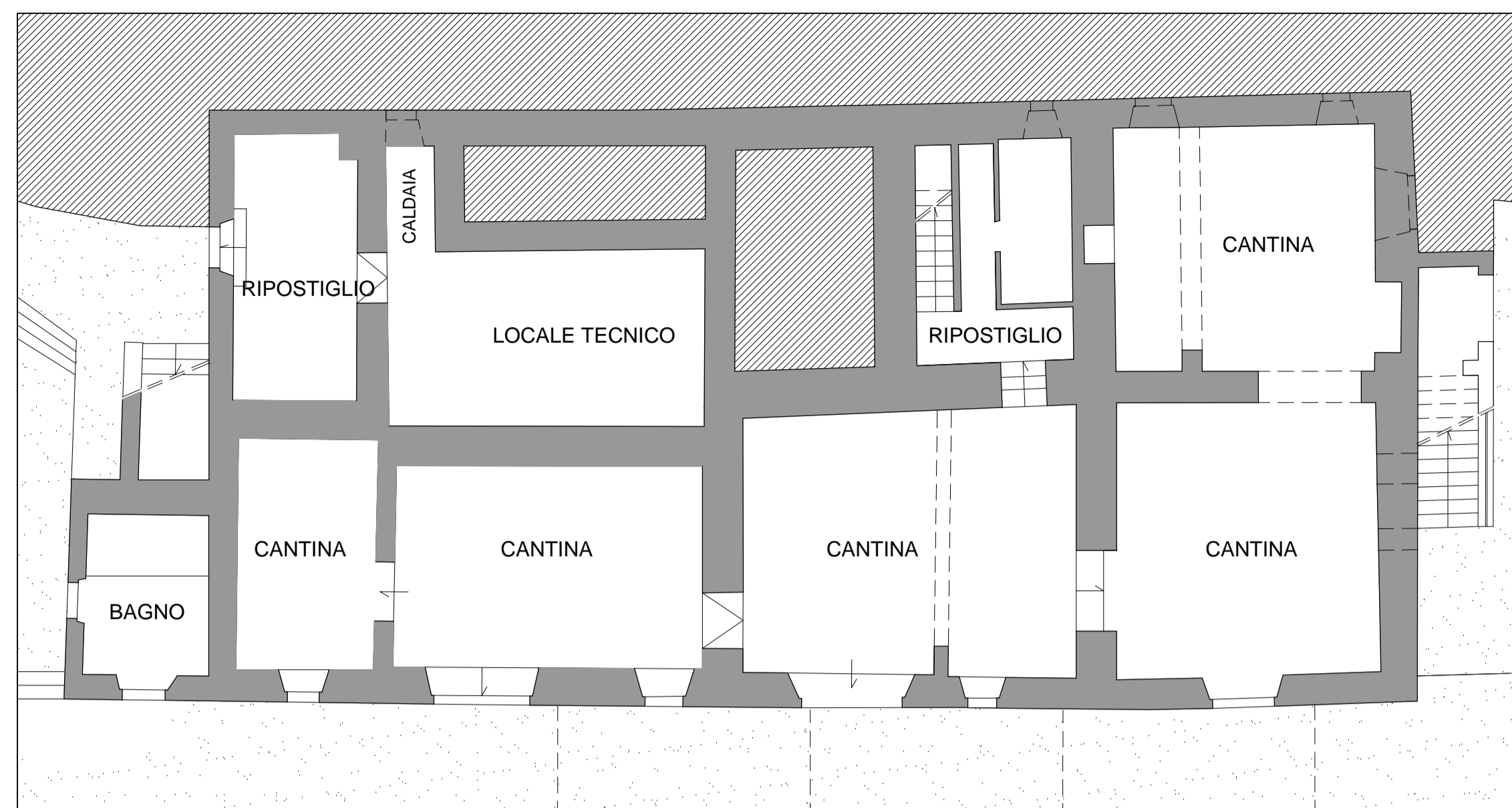
PIANTA PIANO CANTINA - STATO DI FATTO SCALA 1:100
