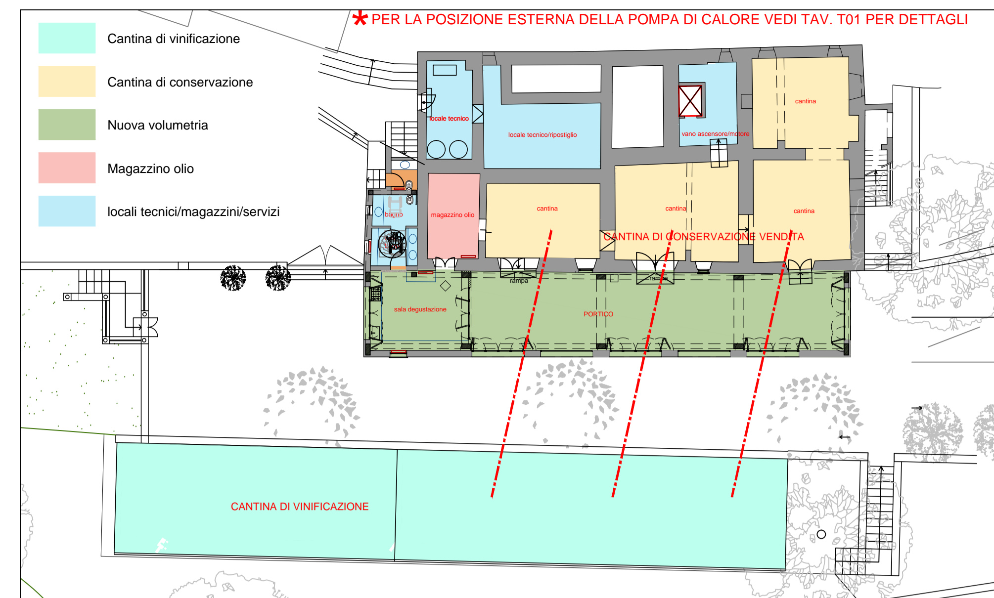
PLANIMETRIA - POSIZIONE SCHEMATICA DI TRE TUBAZIONI IN ACCIAIO DIAM. 10-12 INTERRATE DI COLLEGAMENTO TRA LA CANTINA DELLA VINIFICAZIONE E LA CANTINA DI CONSERVAZIONE SCALA 1:200
