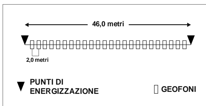
Fig.2.1 - Schema sismica a rifrazione e MASW
